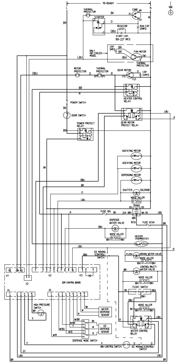
DCM-750BAH-OS, DCM-750BWH-OS
